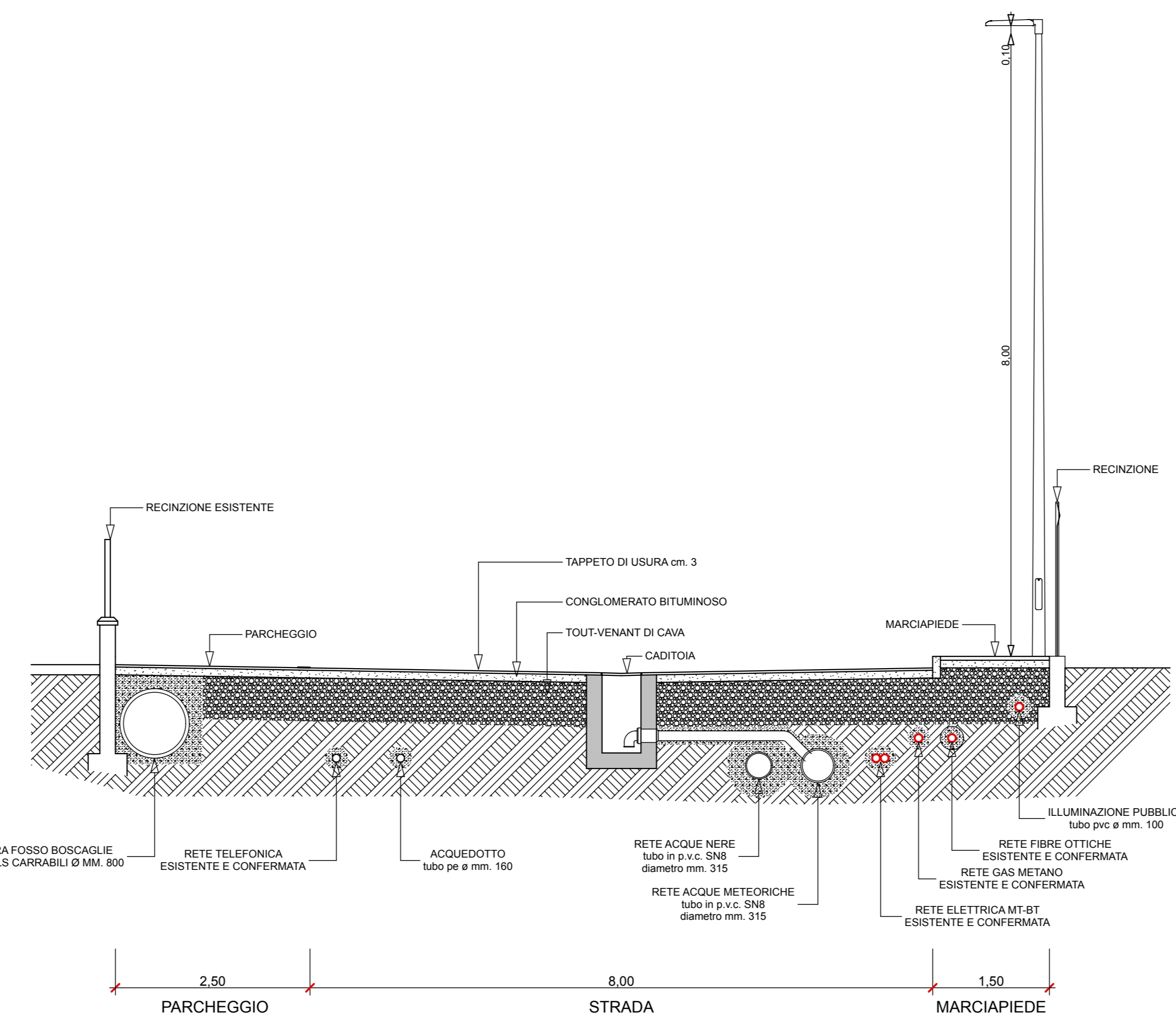
SEZIONE A-A
