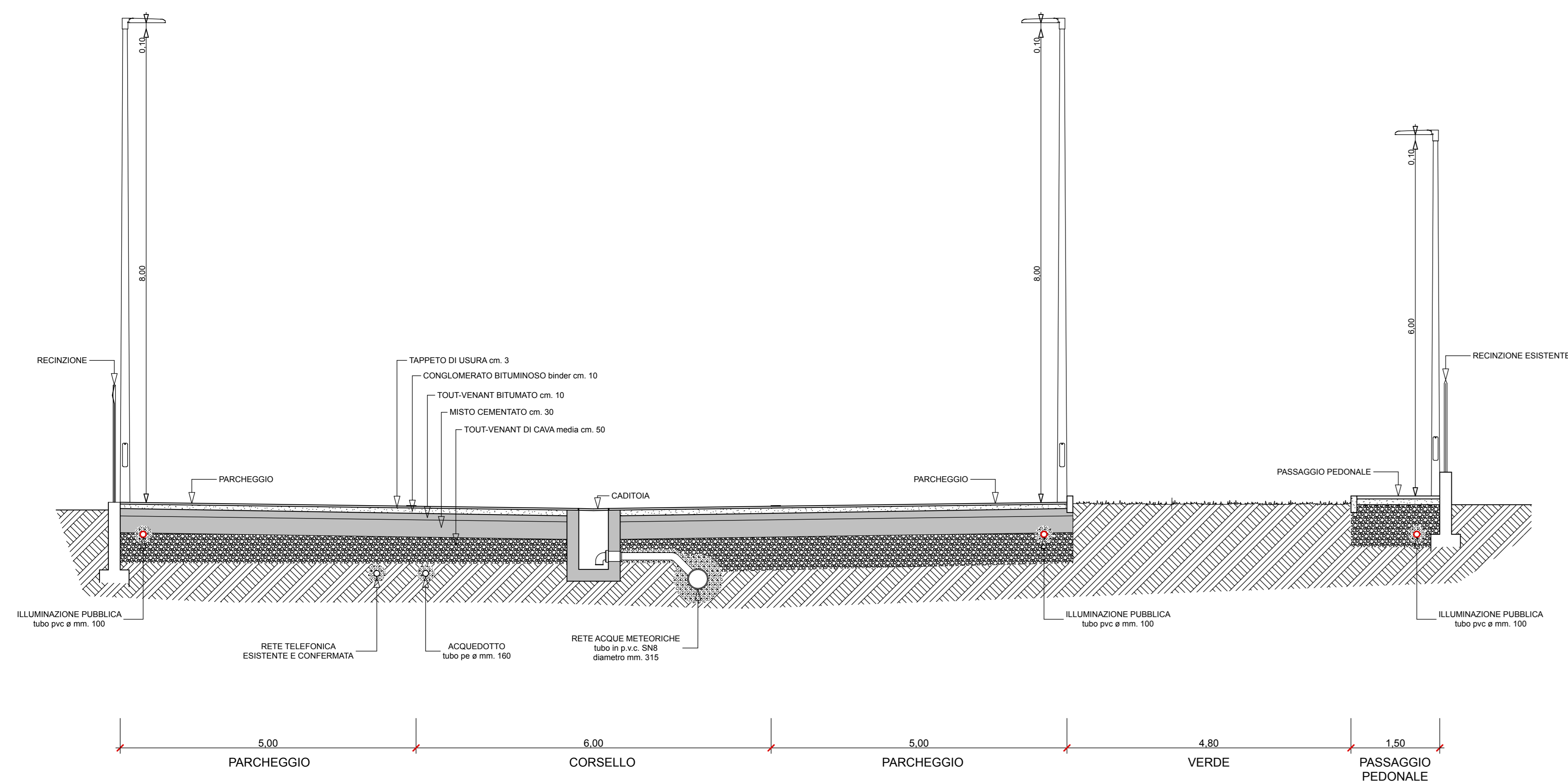
SEZIONE B-B
